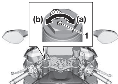
1. 快速壓縮減震力調整器
