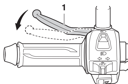
1. 後煞車把手
