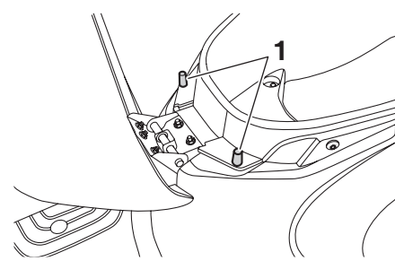
1. 安全帽掛鉤
