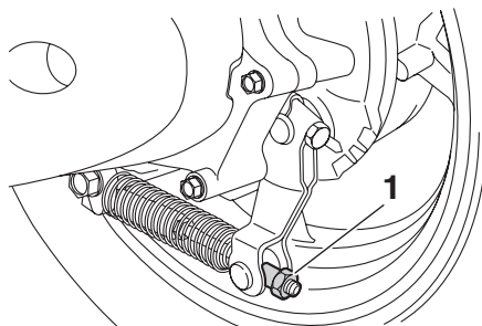
1. 調整螺帽 (請勿自行旋轉)
