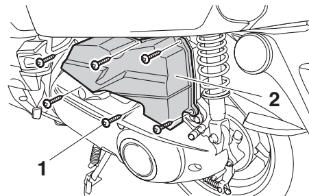
1. 螺絲(x6) 2. 空氣濾清器蓋
