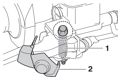
1. 樞軸 2. 橡皮套
