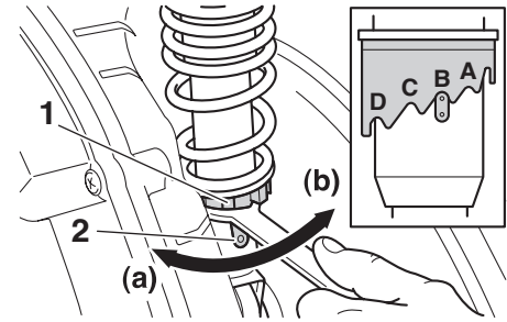
1. 調整環 2. 位置指示器
