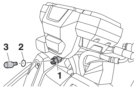
1. 燈泡固定座 2. 密封環 3. 燈泡
