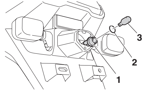
1. 燈泡固定座 2. 密封環 3. 燈泡
