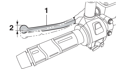
1. 後煞車把手 2. 自由間隙
