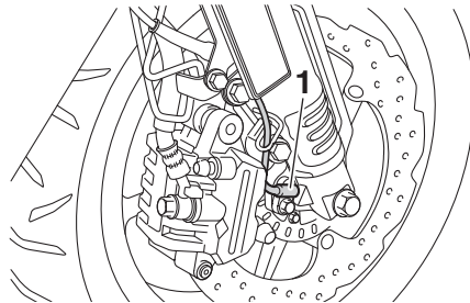
1. 前輪感知器
