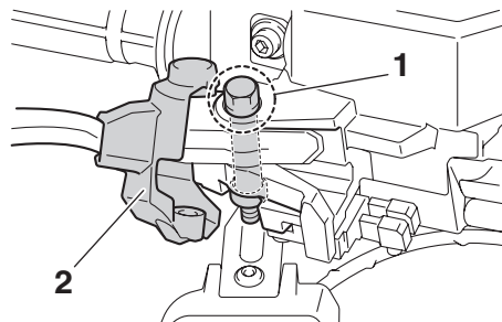
1. 樞軸 2. 橡皮套
